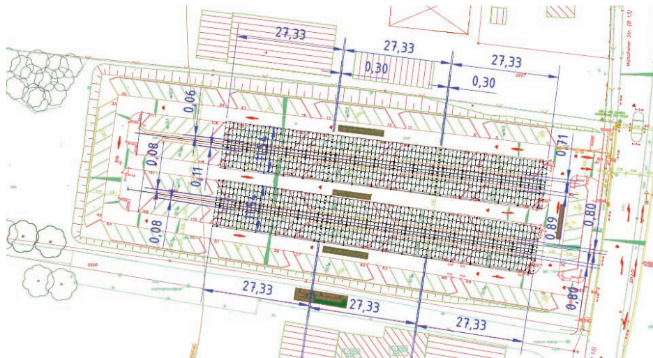
Bild 1: Das Bild zeigt die Planskizze der Photovoltaikanlage am P&R Parkplatz Bahnhof Pfaffenhofen a.d. Ilm.
